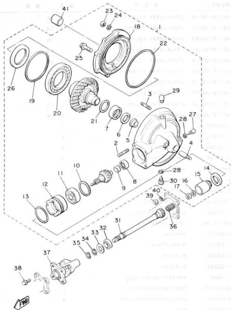
FIG. 26 ト"ライフ"シャフト
