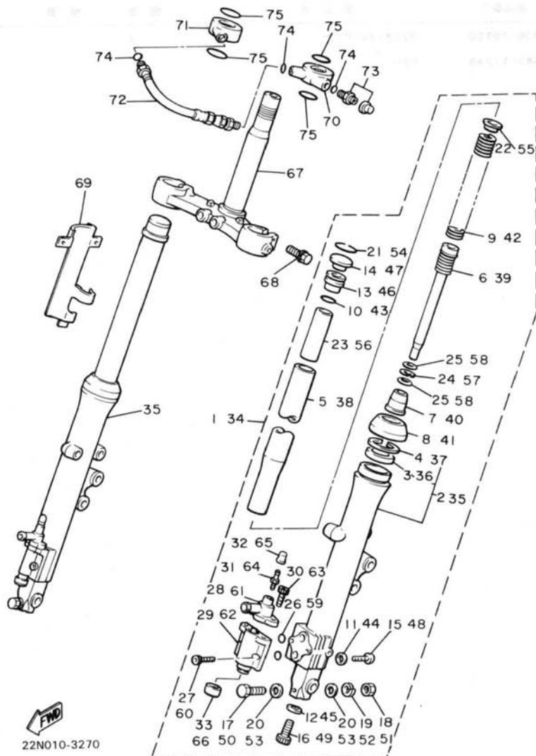
FIG. 27 フロントフォーク
