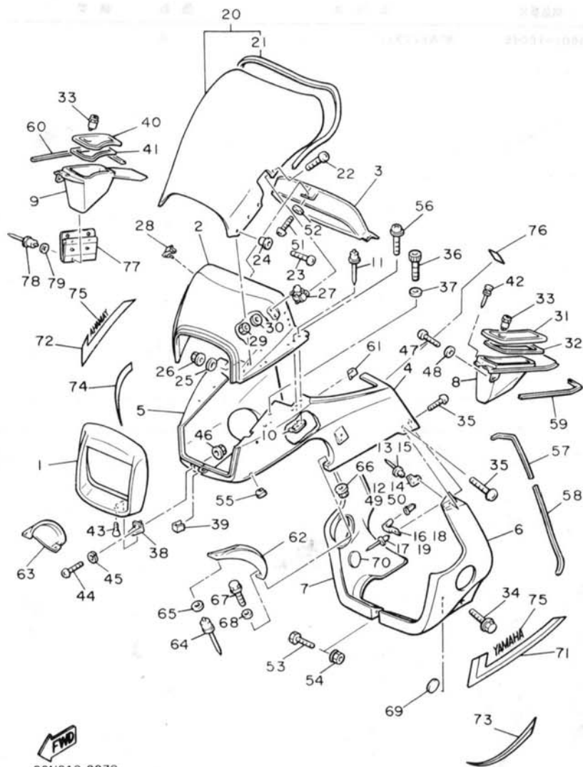
FIG. 37 カウリング 1
