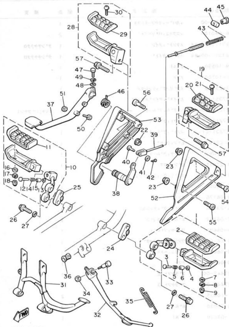
FIG. 36 スタント・フートレスト
