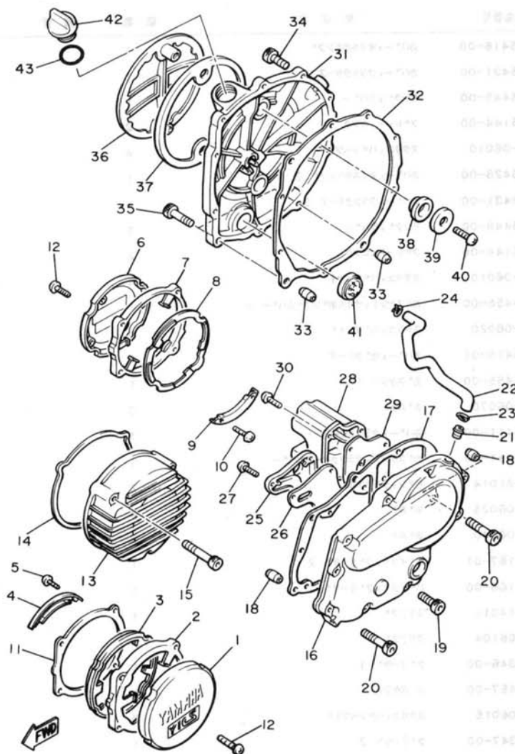
FIG. 12 クランクケースカバー
