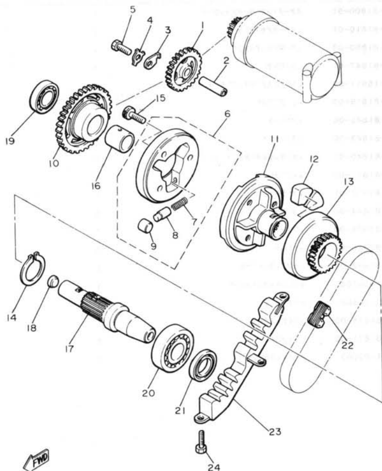
FIG. 16 スタータクラッチ
