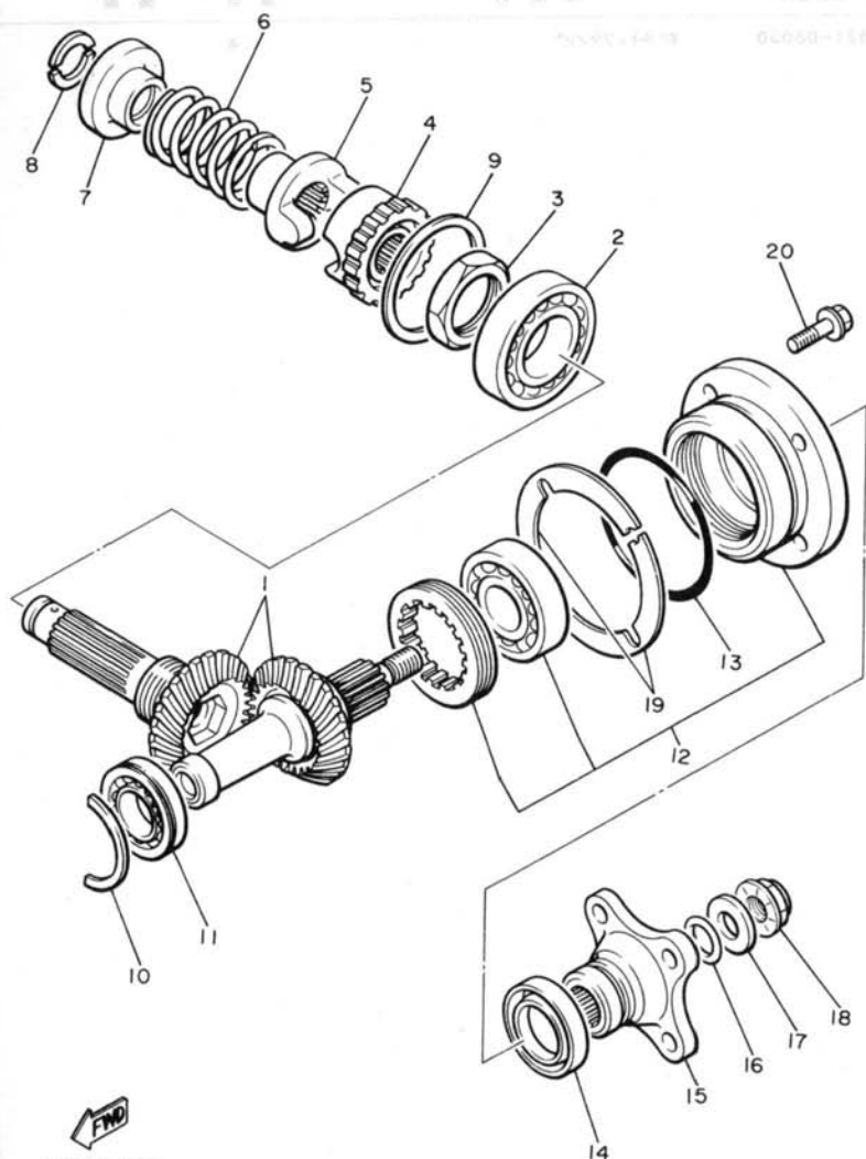
FIG. 19 ミト"ルト"ライフ"キ"ヤ
