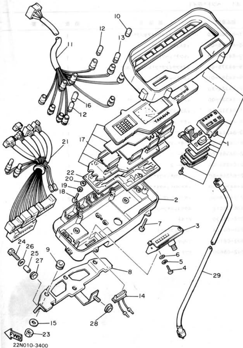
FIG. 40 メータ
