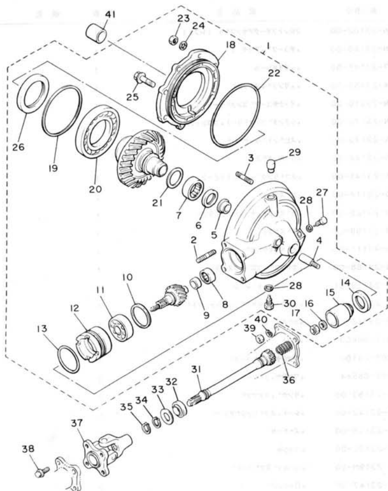
FIG. 26 トライフシャフト
